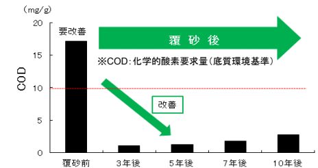
図3 覆砂による底質改善効果
